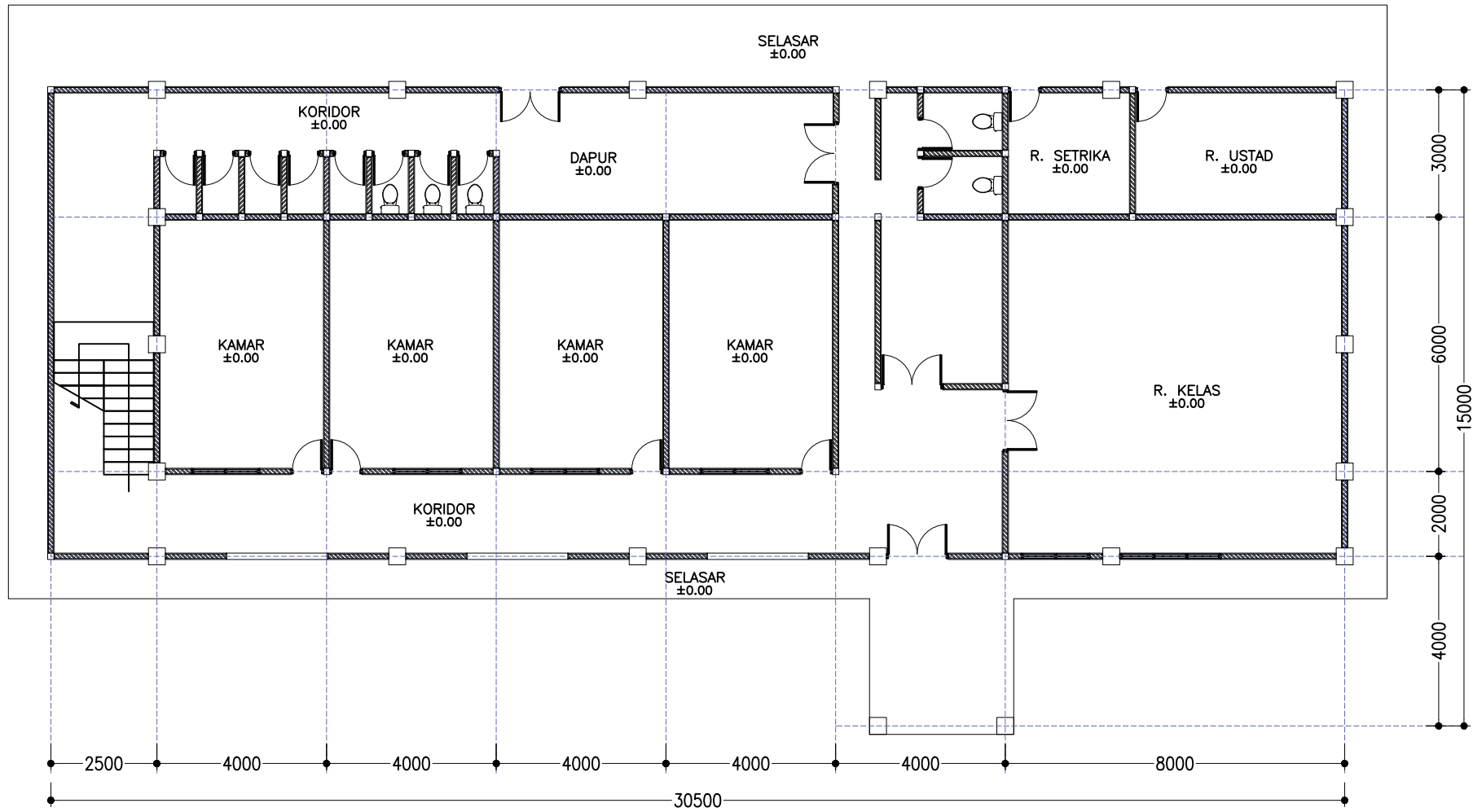
DENAH LT.1 1:100
