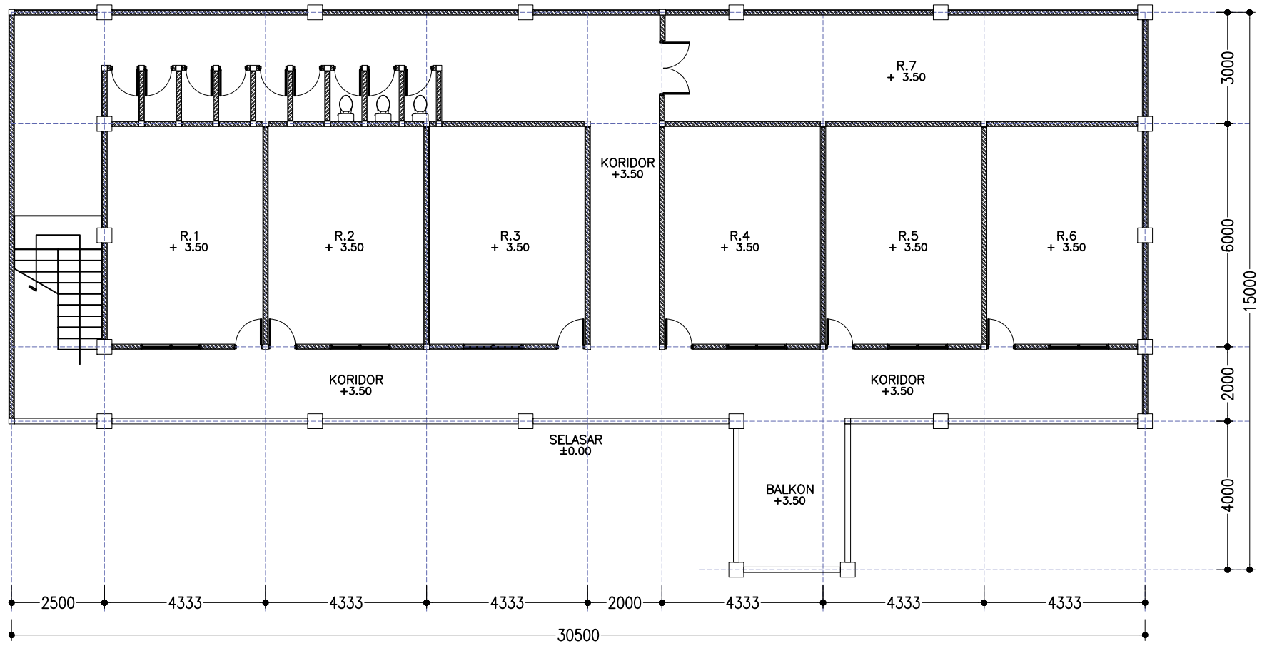
DENAH LT.2 1:100
